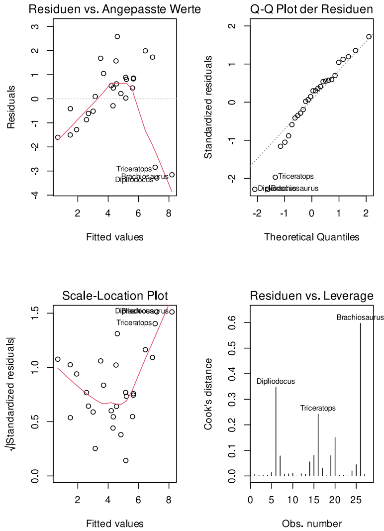
Abbildung 1: Diagnostische Plots für die Regressionsanalyse
