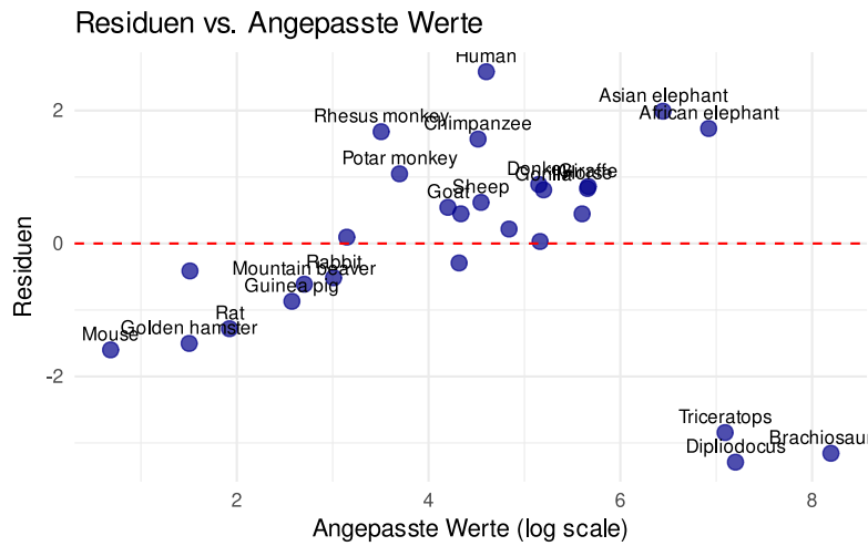
Abbildung 1: Residuen der logarithmischen Regression zur Identifikation von Ausreissern
